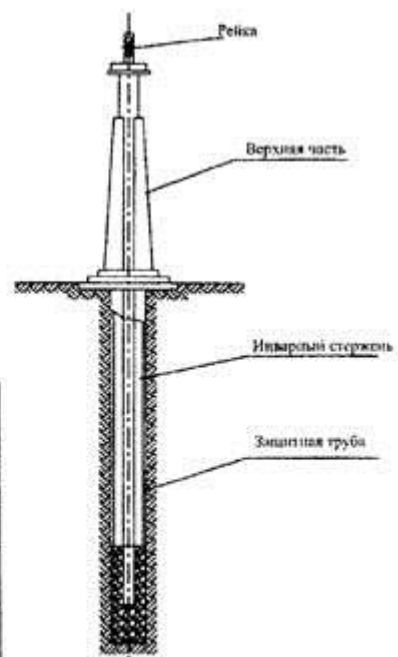
Глубинный репер
