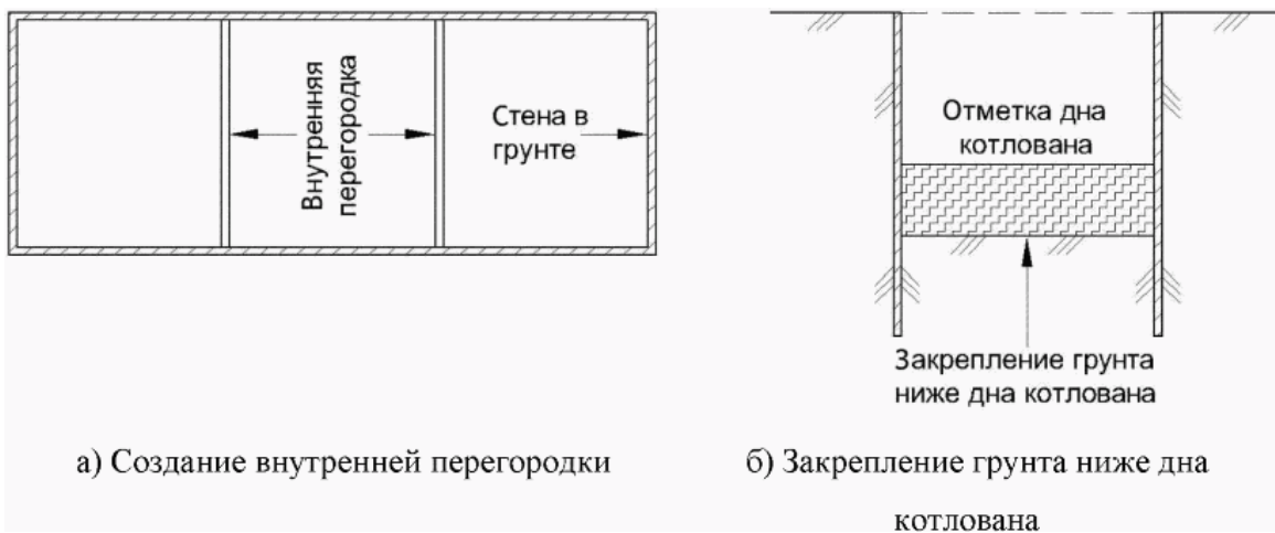
Рисунок 8.1 - Повышение жесткости удерживающей системы ограждающей конструкции
